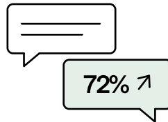
Sycophancy
